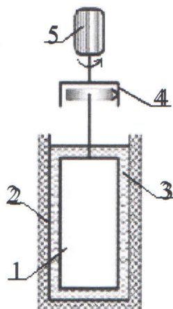
Рисунок 1 - Принципиальная схема ротационного вискозиметра 1 - шпindel, 2 - сосуд, 3 - проба вязущего; 4 - измерительный механизм, 5 – двигатель
